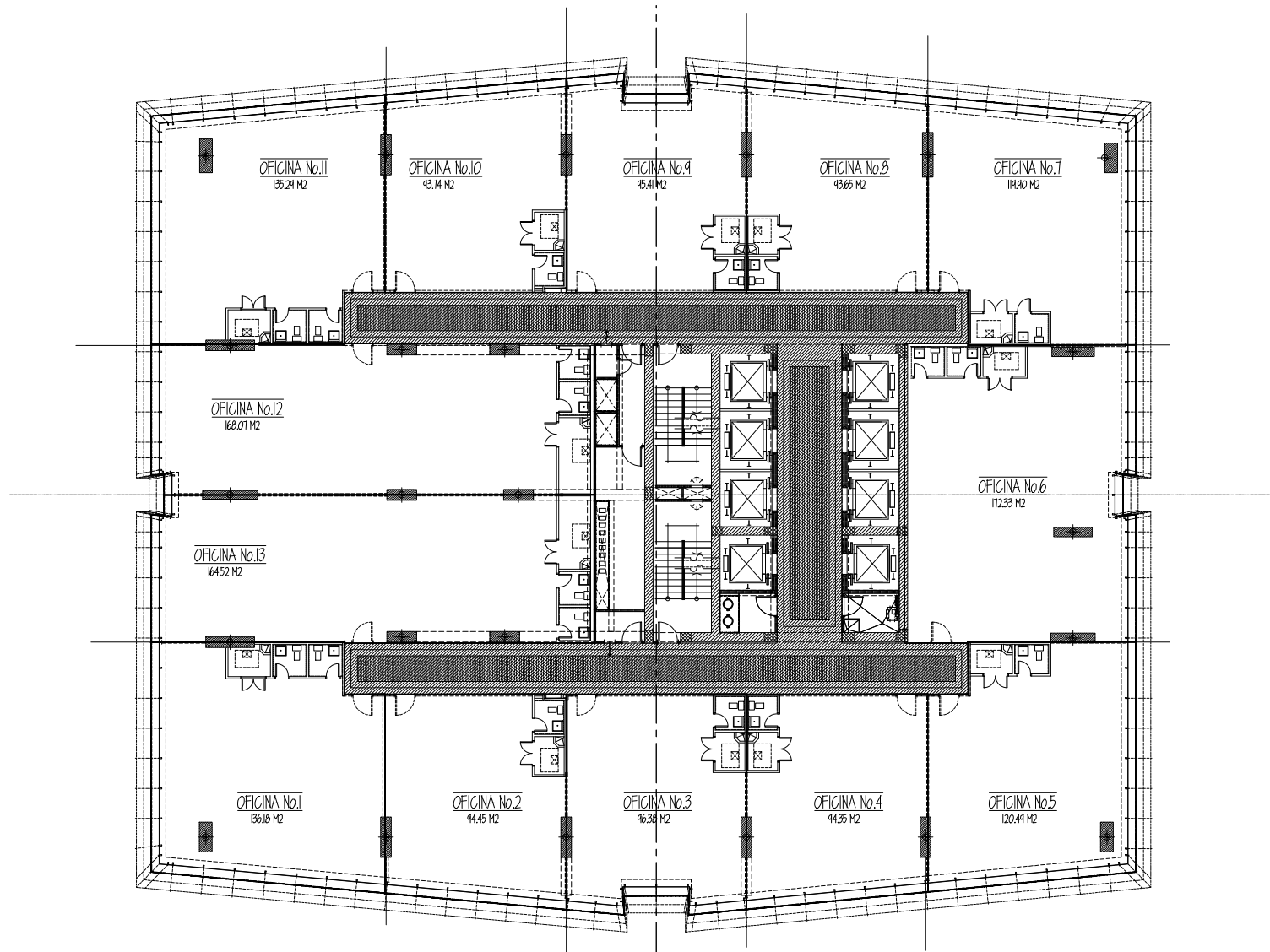
PLANTA DE ARQUITECTURA - NIVEL 4100.00 ESCALA 1:100 OFICINAS
