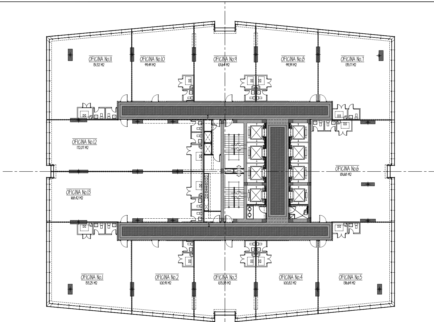
PLANTA DE ARQUITECTURA - NIVEL 4000.00 ESCALA 1:100 OFICINAS
