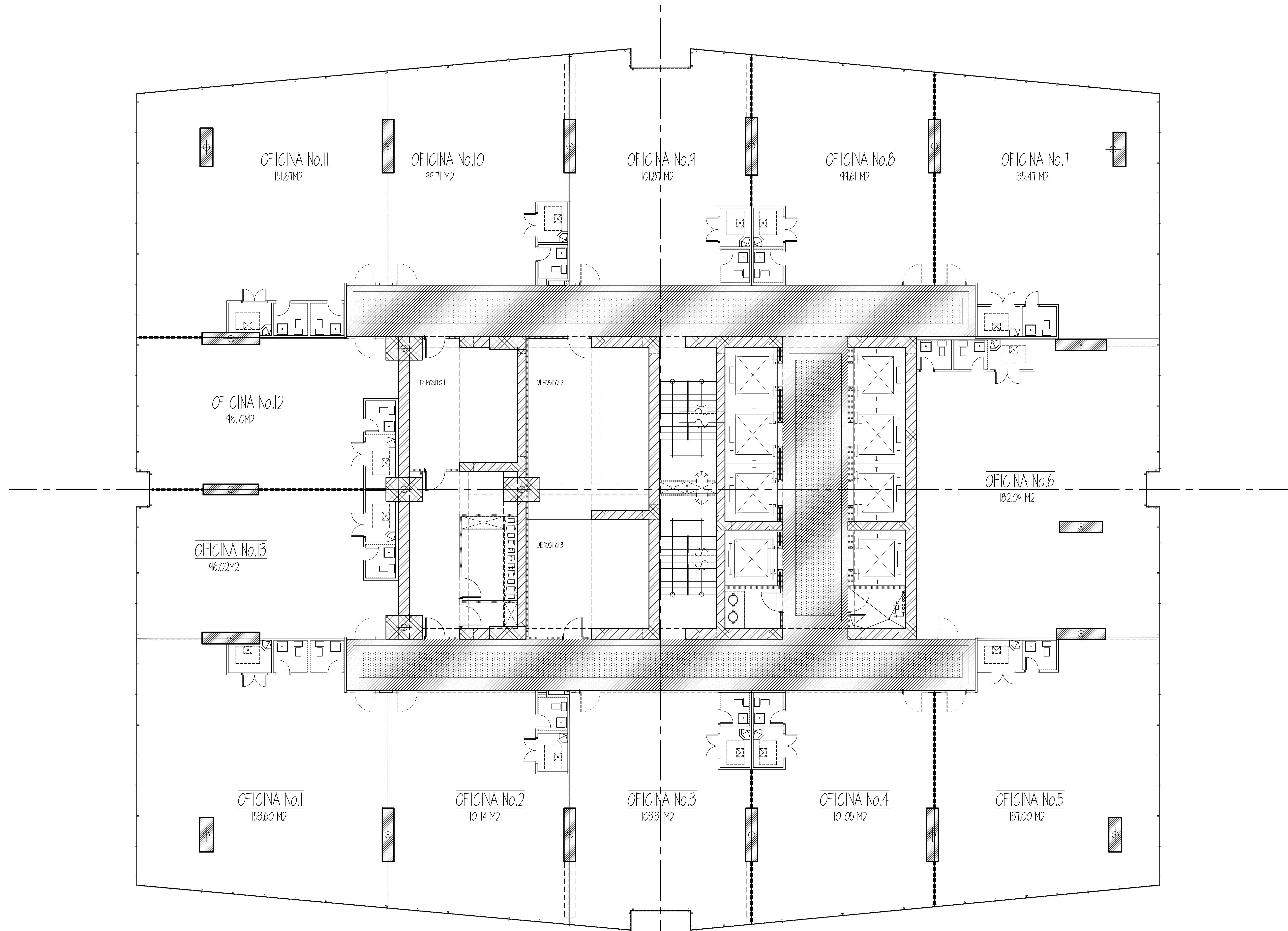
PLANTA DE ARQUITECTURA - NIVEL 2600.00 ESCALA 1:100 OFICINAS
